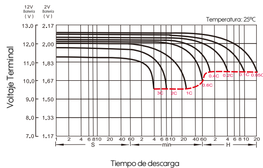
Características de descarga a 25 °C
